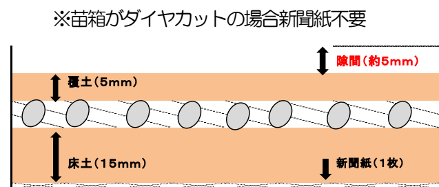
■図1：播種後の苗箱断面図
