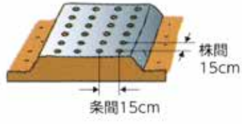
図2 トンネルの設置
